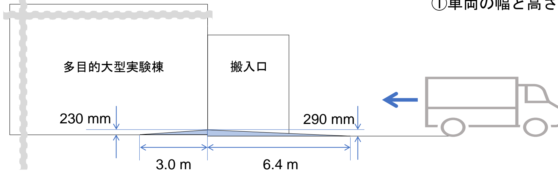
②傾斜 車体と地面とのクリアランス
